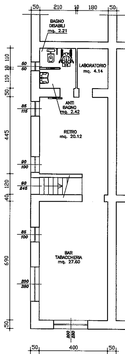
PIANTA PIANO TERRA STATO DEFINITIVO
