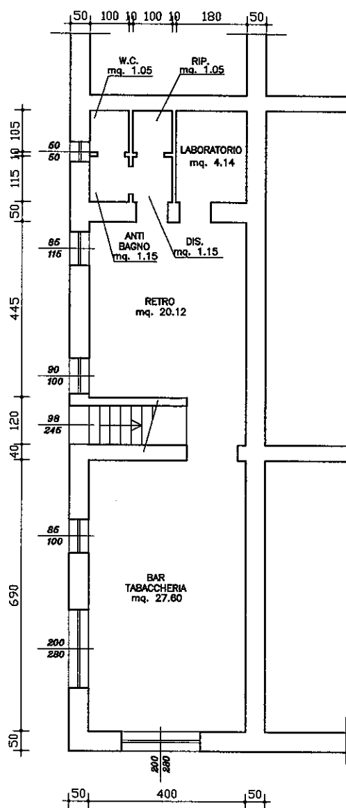
PIANTA PIANO TERRA STATO ATTUALE
